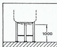
Stålstativ
